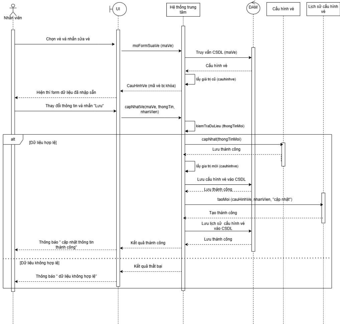
Image 7: Sơ đồ tuần tự sửa vé
