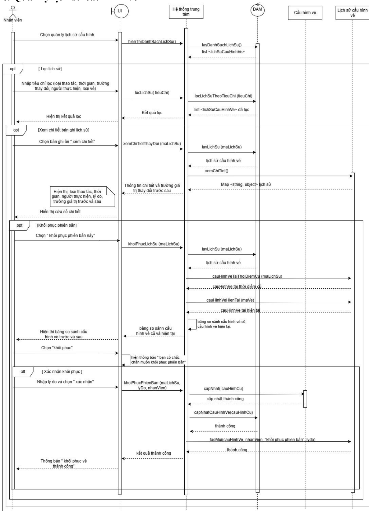
Image 9: Sơ đồ tuần tự quản lý lịch sử cấu hình vé
